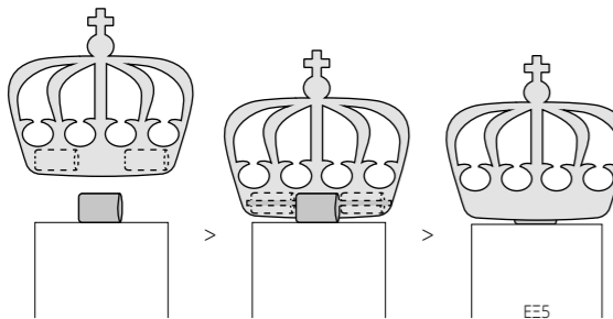
ΕΞ5 Μικρός κύλινδρος, συγκολλημένος στο κέντρο του πάνω μέρους του σταυρού, προσαρμόζεται ανάμεσα σε δύο όμοιους κρυφούς κυλίνδρους συγκολλημένους εσωτερικά στο στέμμα. Τους τρεις κυλίνδρους διαπερνά άξονας.
