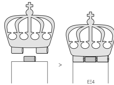
ΕΞ4 Μικρός, ενιαίος κύλινδρος, συγκολλημένος στο κέντρο του πάνω μέρους του σταυρού, προσαρμόζεται ανάμεσα σε δύο παρόμοιους κυλίνδρους στο κάτω μέρος του στέμματος. Τους τρεις κυλίνδρους διαπερνά άξονας.
