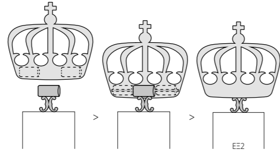
ΕΞ2 Έλασμα σε σχήμα Χ, συγκολλημένο στο πάνω μέρος του σταυρού, απολήγει σε μικρό κύλινδρο, τον οποίο διαπερνά άξονας συγκολλημένους εσωτερικά στο στέμμα του σταυρού.
