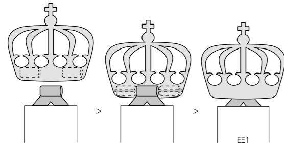
ΕΞ1 Έλασμα σε σχήμα Λ, συγκολλημένο στο πάνω μέρος του σταυρού, απολήγει σε μικρό κύλινδρο που προσαρμόζεται ανάμεσα σε δύο όμοιους κρυφούς κυλίνδρους συγκολλημένους εσωτερικά στο στέμμα, απ' όπου περνά άξονας.
